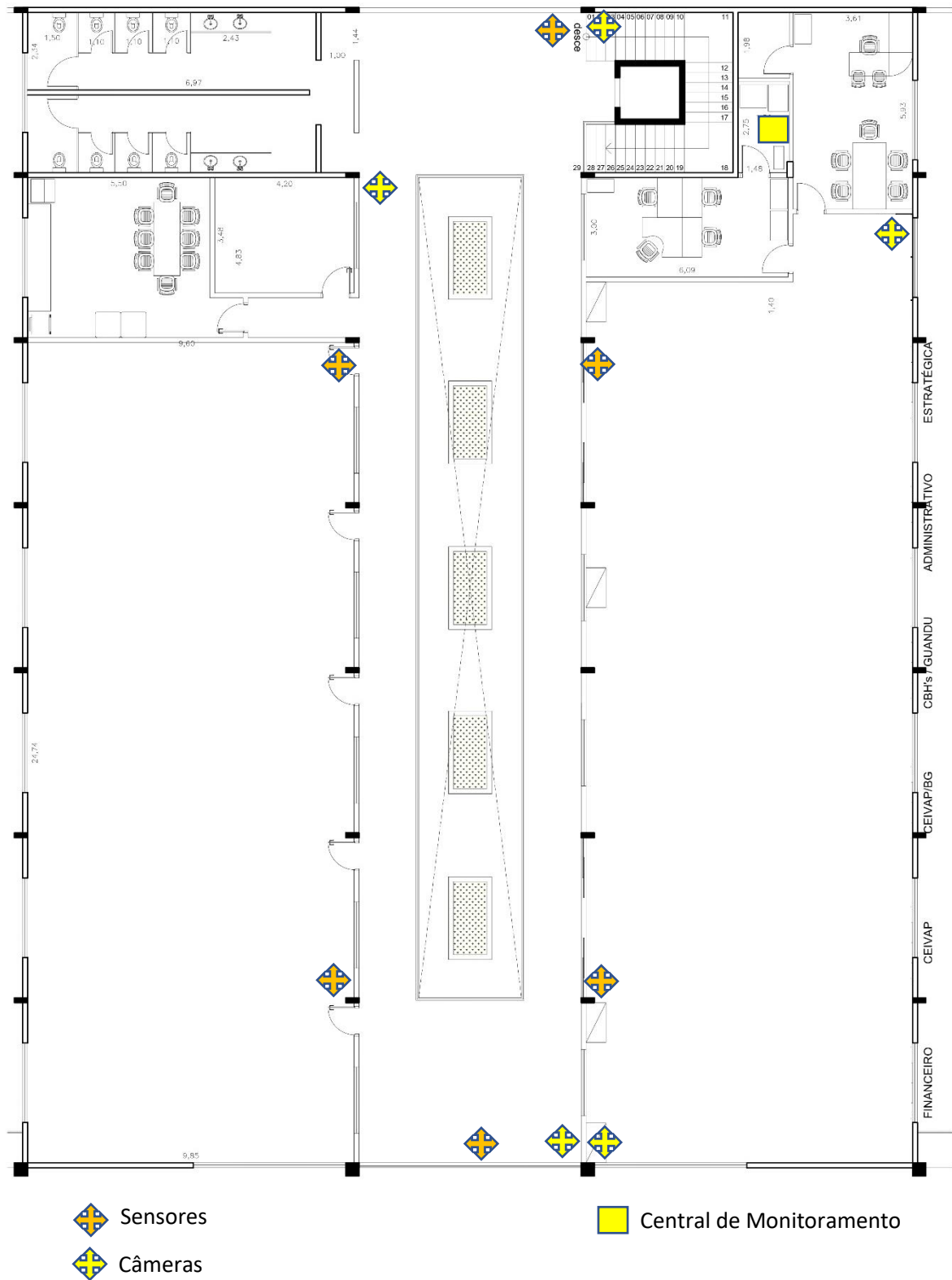
Figura 12-Layout posicionamento Câmeras e Sensores
