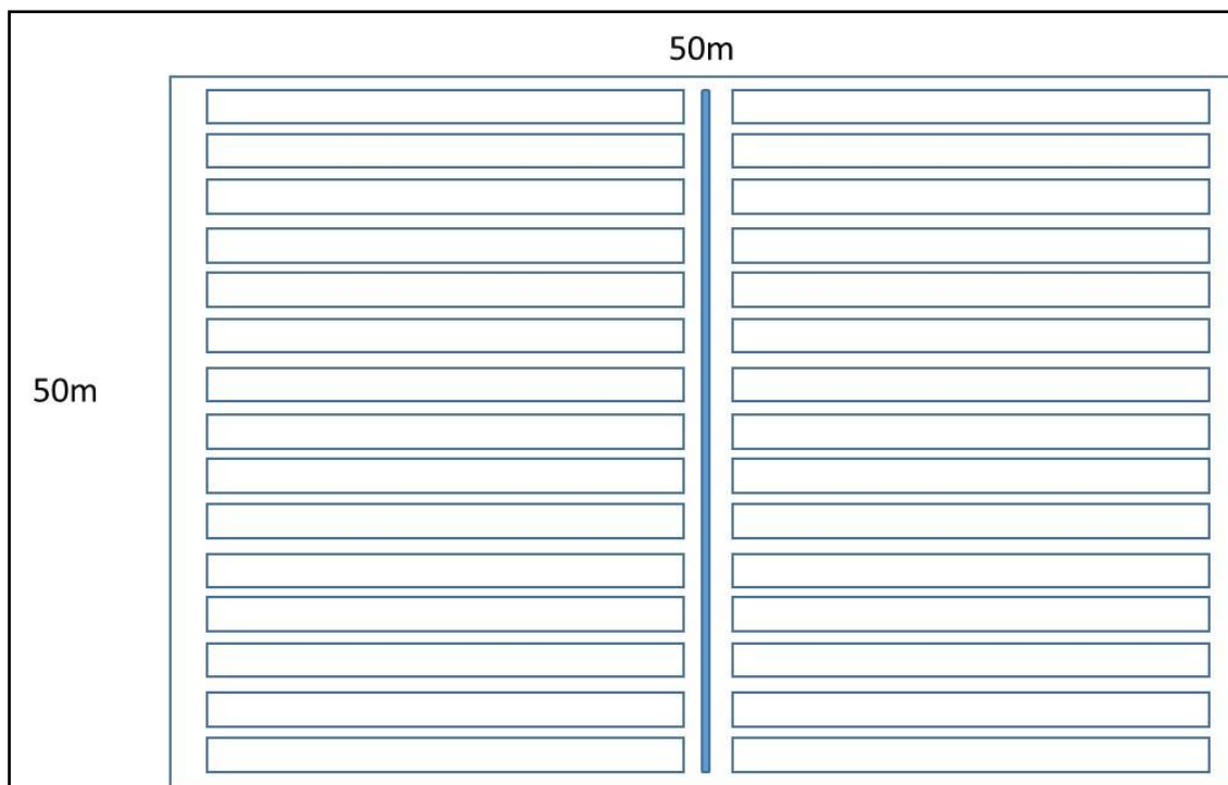
Figura 6 – Layout do kit de irrigação por gotejamento
