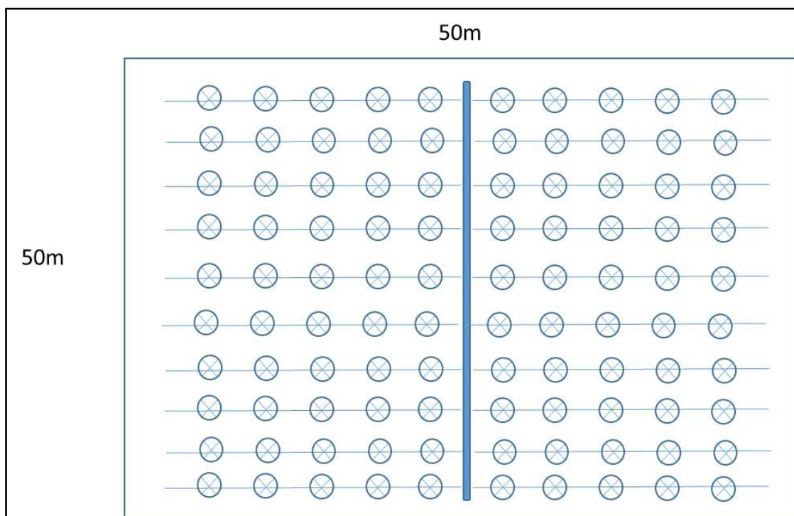
Figura 5. Layout do kit de irrigação por microaspersão.
