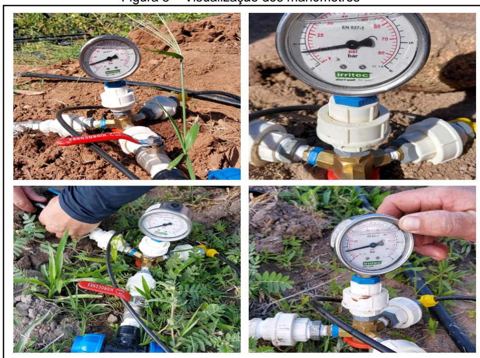
Figura 5 – Visualização dos manômetros
